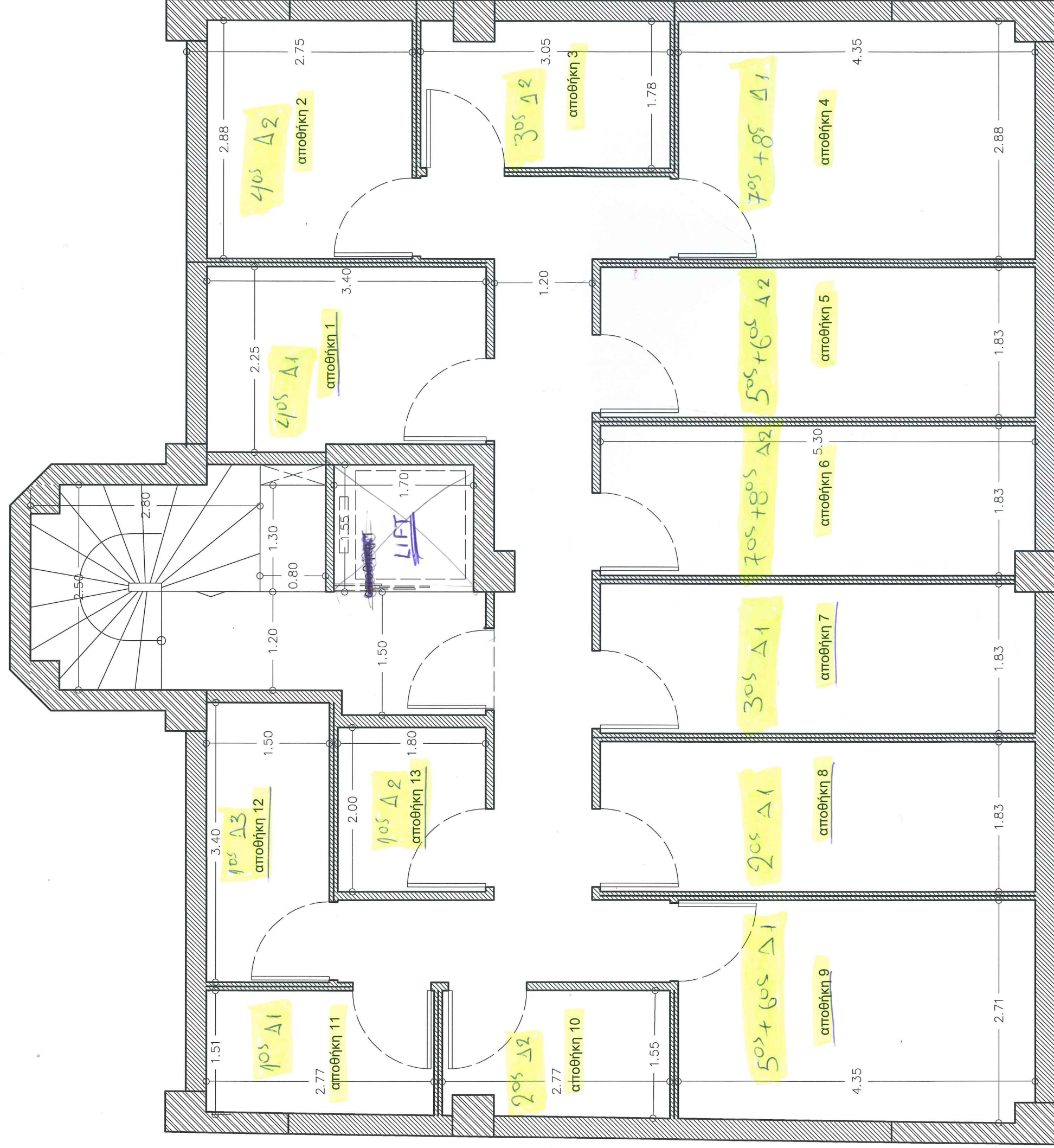
ΙΩΑΝΝΗ ΓΚΟΥΡΑ 15 ΚΑΤΟΨΗ ΥΠΟΓΕΙΟΥ
